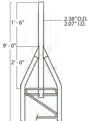
TOP SECTION 45AG2
